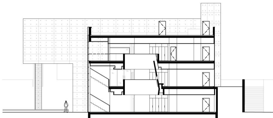
D-D SEC
