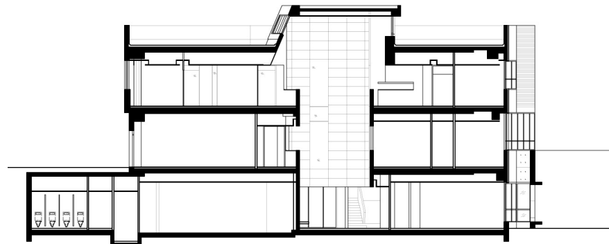
A-A SEC
